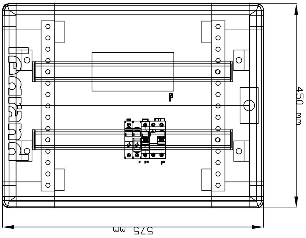
rozdzielnica RF
