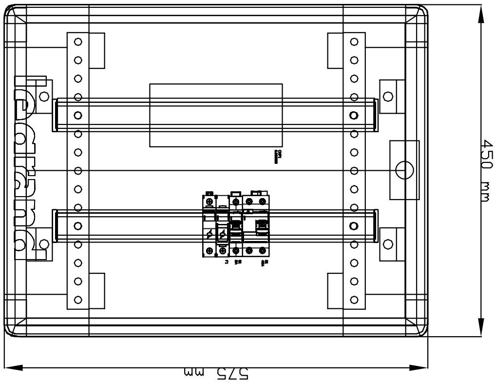
rozdzielnica RF
