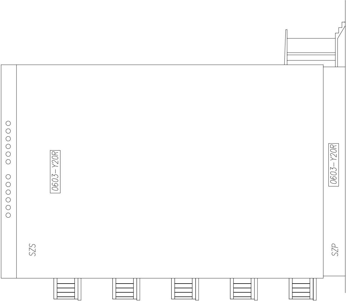
ELEWACJA POŁUDNIOWA
